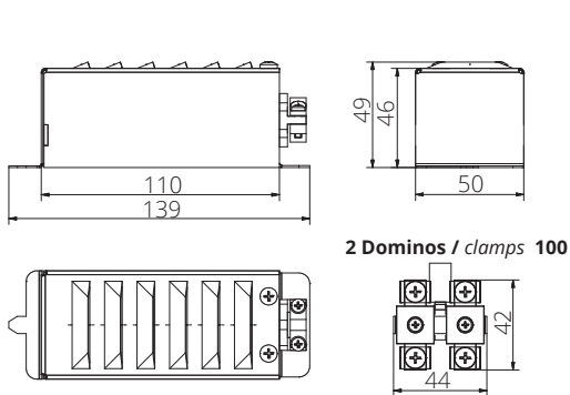
Connecteur à câble type KA150 KA150 cable fitting
