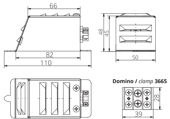
Connecteur à câble type KA155 KA155 cable fitting
