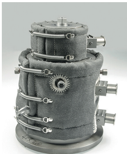
outillage avec isolation tool with insulation, after
